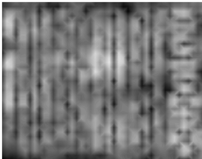
Abbildung 4 : Schwingungsbild der Holzständerwand als Falschfarbenbild (hell hoher Pegel L_a , dunkel niedriger Pegel L_a ) Frequenz f = 346 - 351 Hz, Oberschwingung im Gefach n=3, m=1 , nach Gleichung 1 Die Lage der Ständer ist durch Balken unterhalb des Schwingungsbilds gekennzeichnet.
